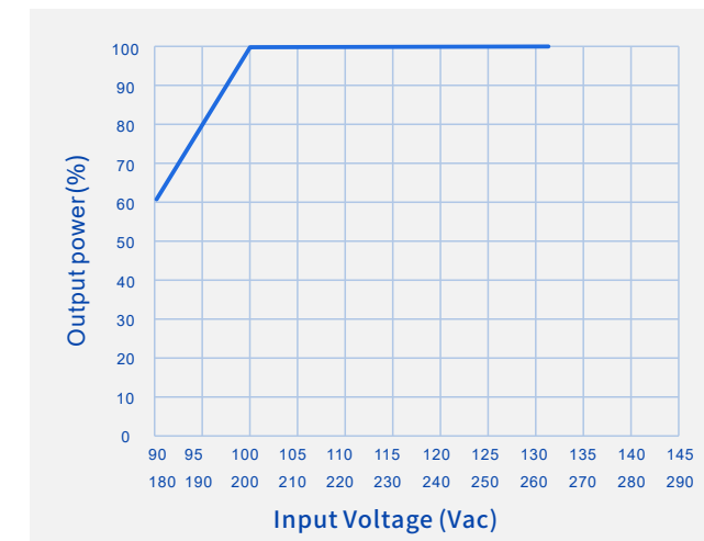
输出功率Vs.输入电压
